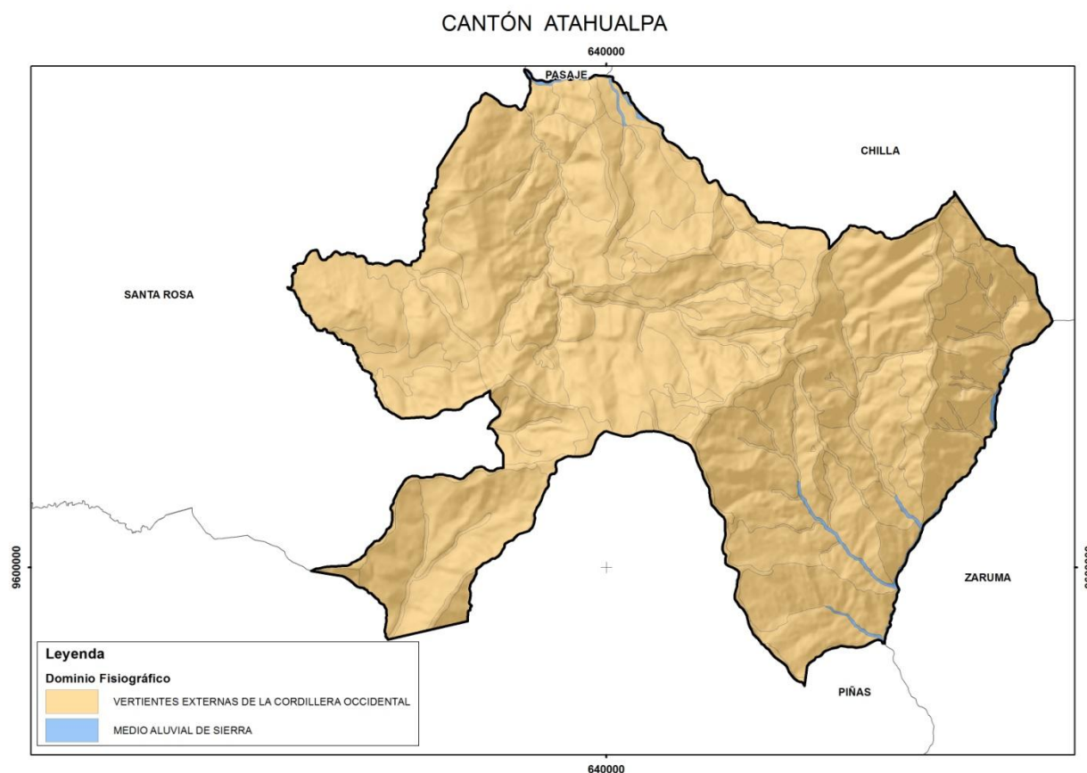
Figura 3.2. Distribución geográfica de los diferentes dominios fisiográficos presentes en el cantón Atahualpa.
