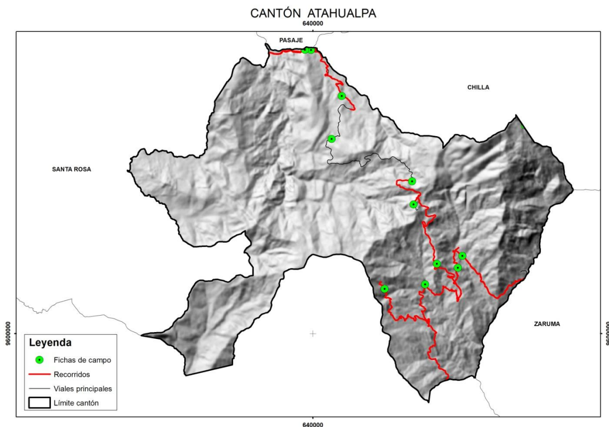
Figura 3.1. Localización de recorridos y fichas de campo del cantón Atahualpa.
