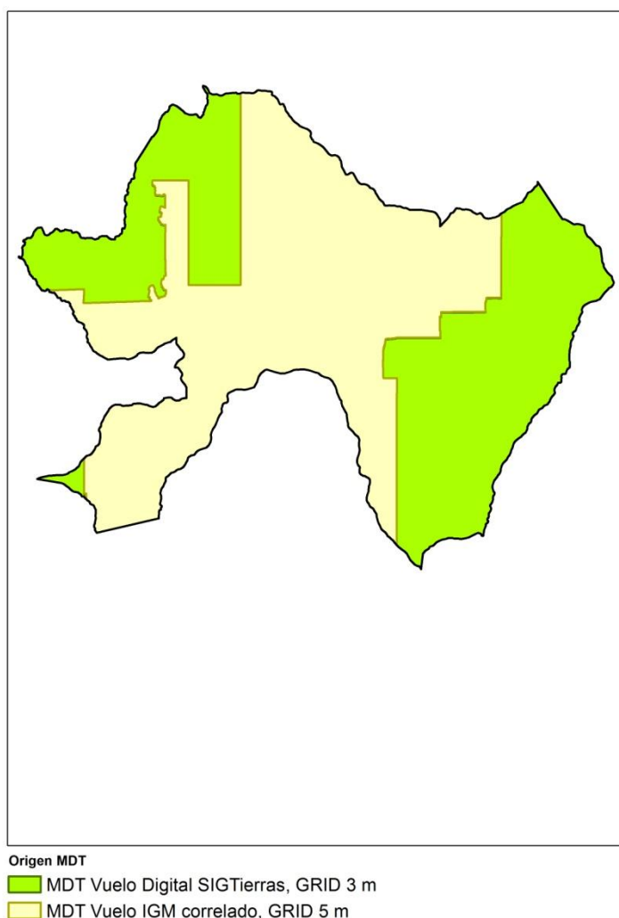
Figura 2.3. Insumos de base de generación de los MDT en el cantón Atahualpa.
