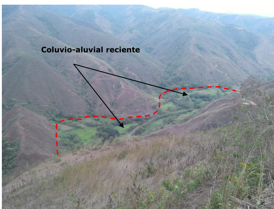
Foto 14. . Sector El Triunfo-Las Colpas. 24/11/2014.
