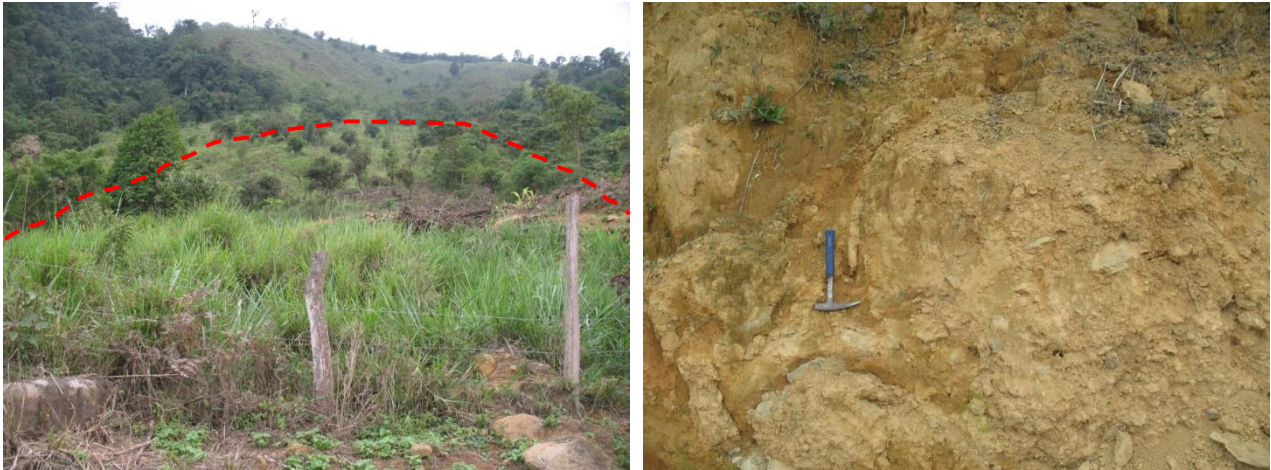
Fotos 9 y 10. Coluvión antiguo. Vista general (izquierda) y detalle del depósito superficial (derecha). Depósitos de ladera (coluvial). Sector Santa Rufina-El Guineo. 04/12/2014.
