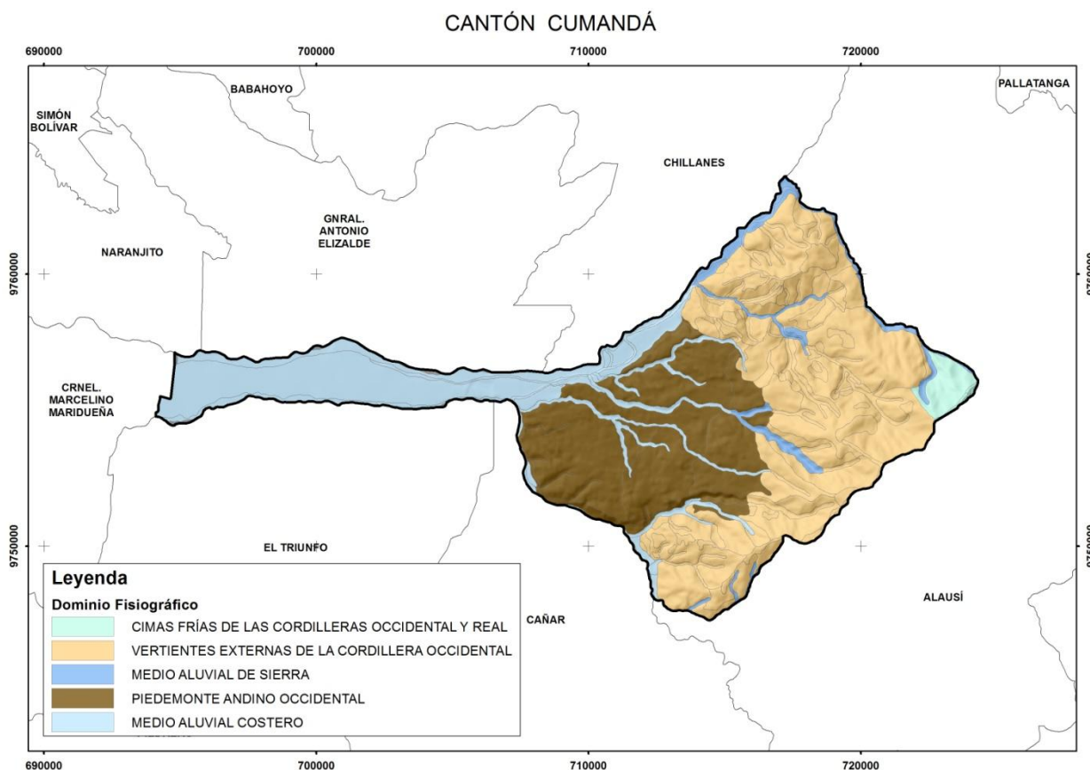
Figura 3.2. Distribución geográfica de los diferentes dominios fisiográficos presentes en el cantón Cumandá.
