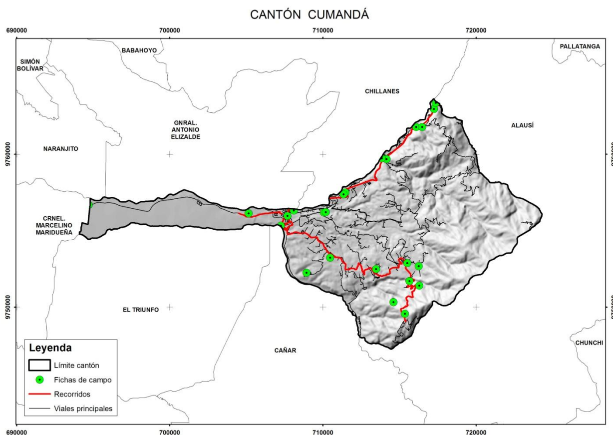
Figura 3.1. Localización de recorridos y fichas de campo del cantón Cumandá.
