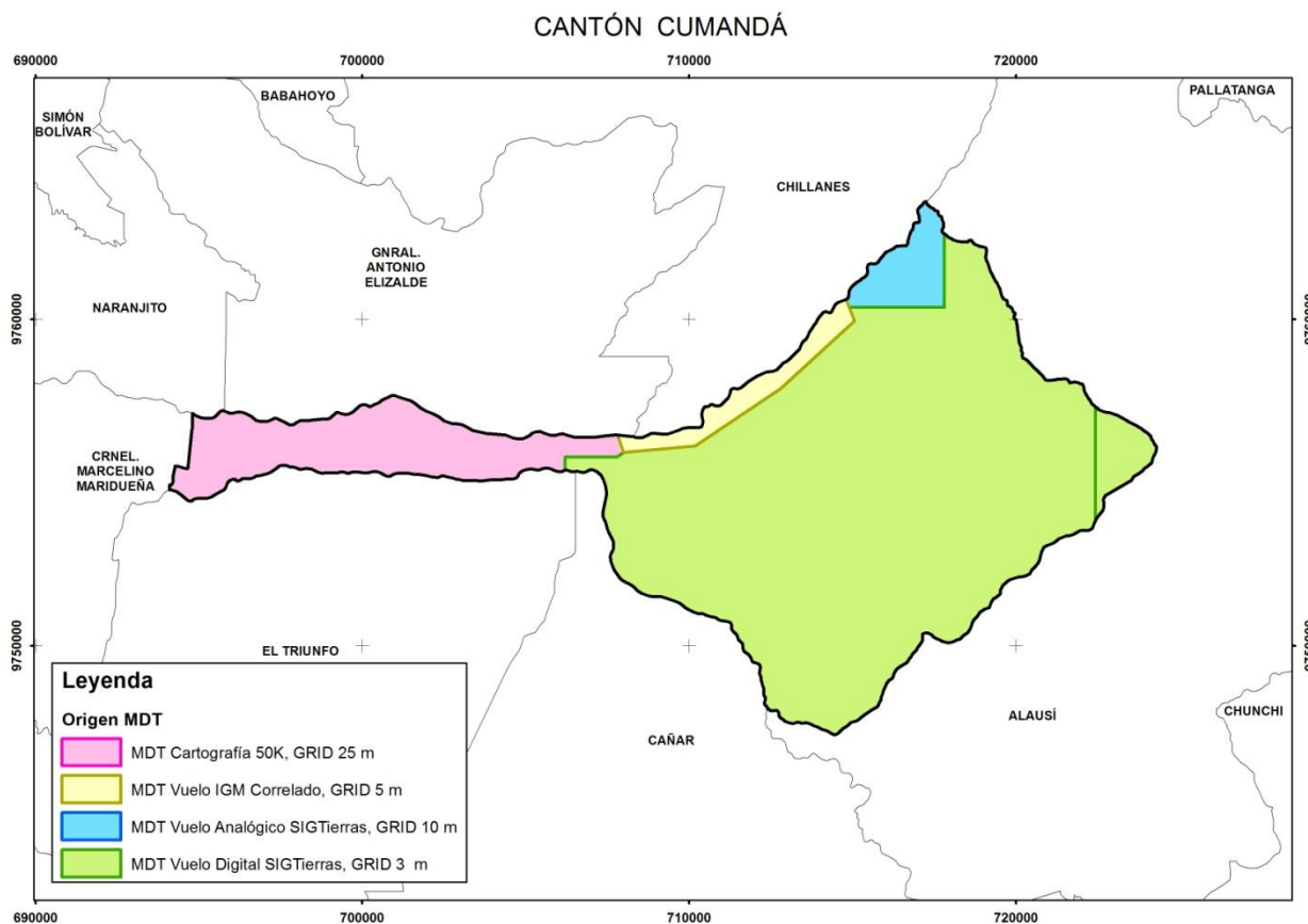
Figura 2.3. Insumos de base de generación de los MDT en el cantón Cumandá.
