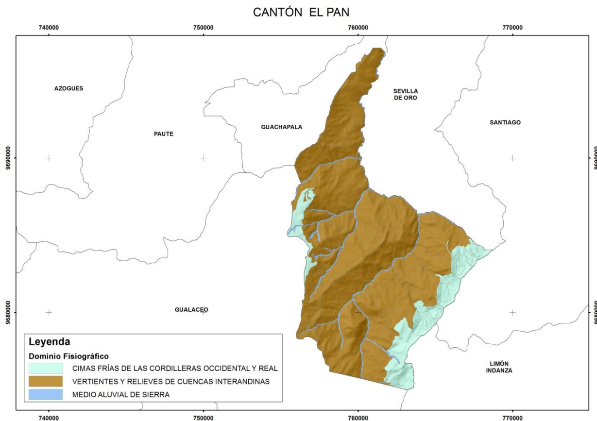
Figura 3.2. Distribución geográfica de los diferentes dominios fisiográficos presentes en el cantón El Pan.
