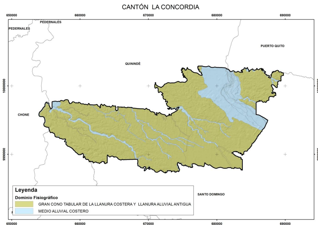
Figura 3.2. Distribución geográfica de los diferentes dominios fisiográficos presentes en el cantón La Concordia.
