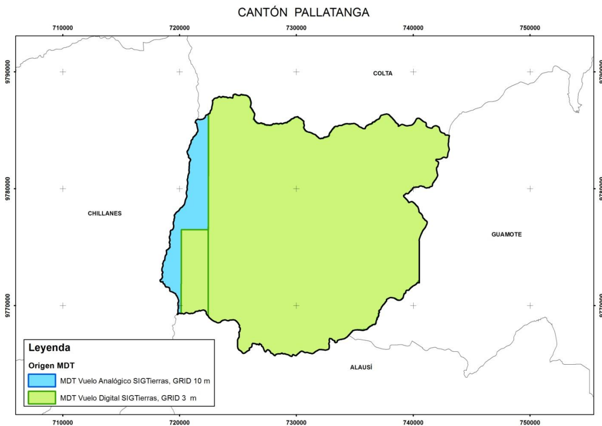
Figura 2.3. Insumos de base de generación de los MDT en el cantón Pallatanga.
