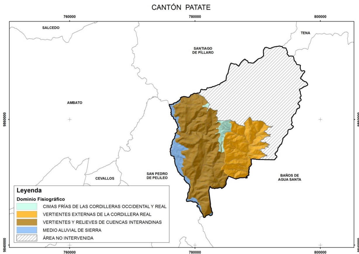
Figura 3.2. Distribución geográfica de los diferentes dominios fisiográficos presentes en el cantón Patate.
