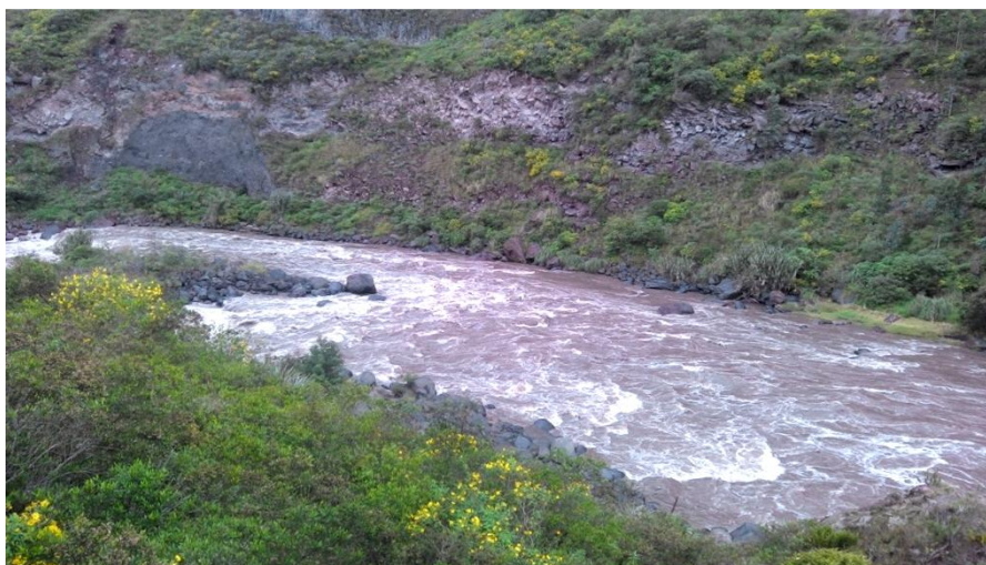
Foto 1. Terraza baja y cauce actual del río Patate, cerca de la confluencia con el río Chambo. 06/06/2014.
