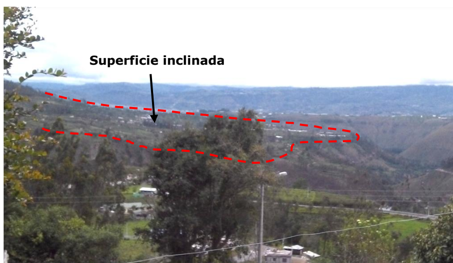
Foto 16. Superficie inclinada, sector Loma Cachourcu. 05/06/2014
