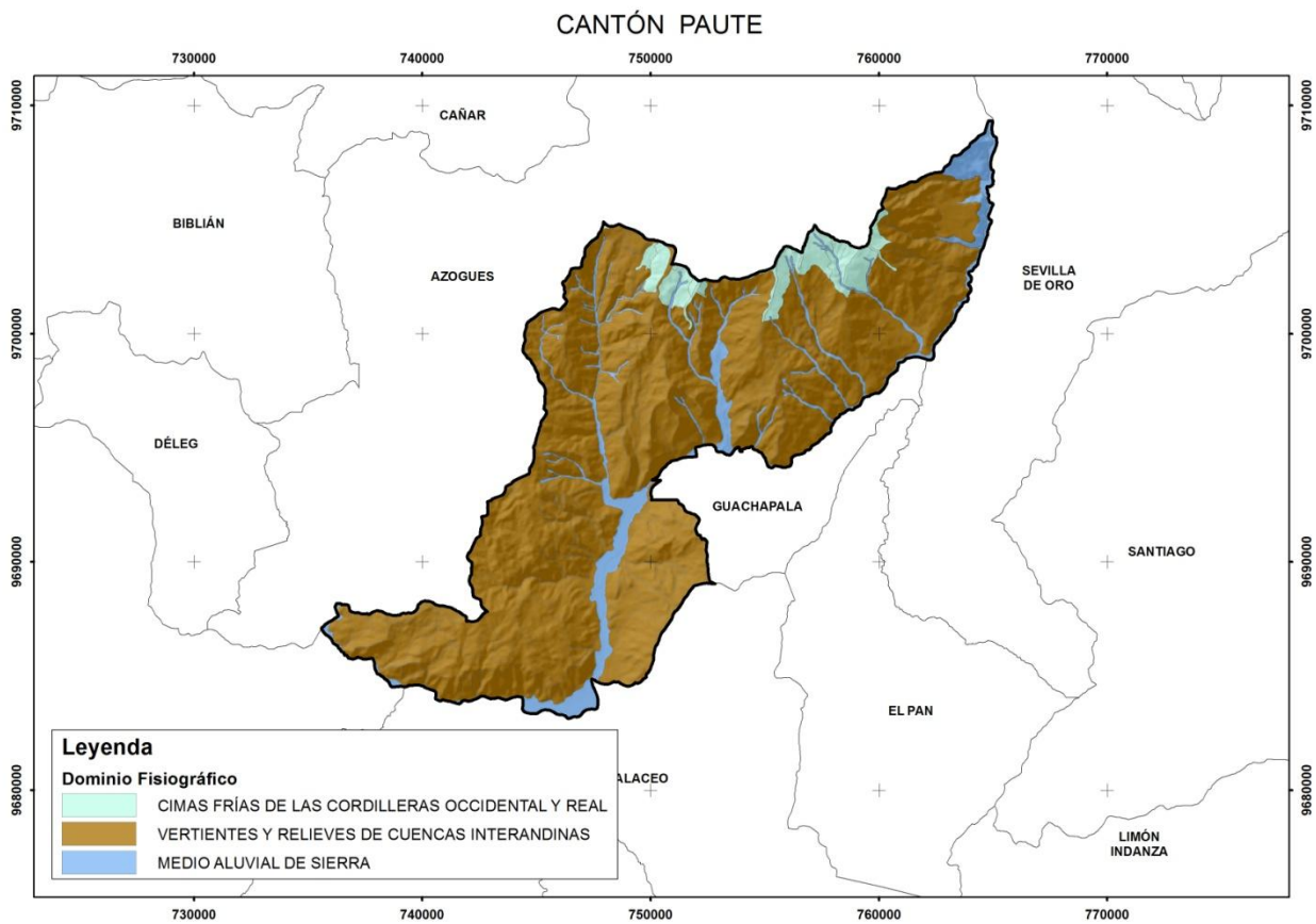
Figura 3.2. Distribución geográfica de los diferentes dominios fisiográficos presentes en el cantón Paute.
