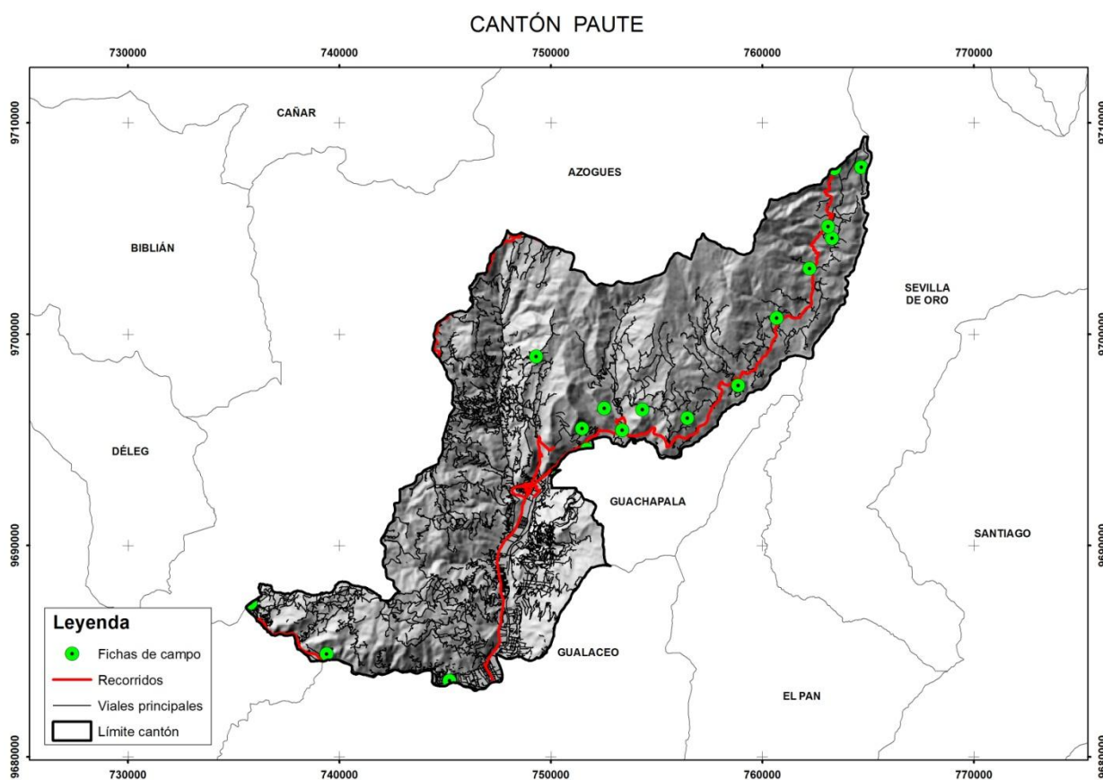
Figura 3.1. Localización de recorridos y fichas de campo del cantón Paute.
