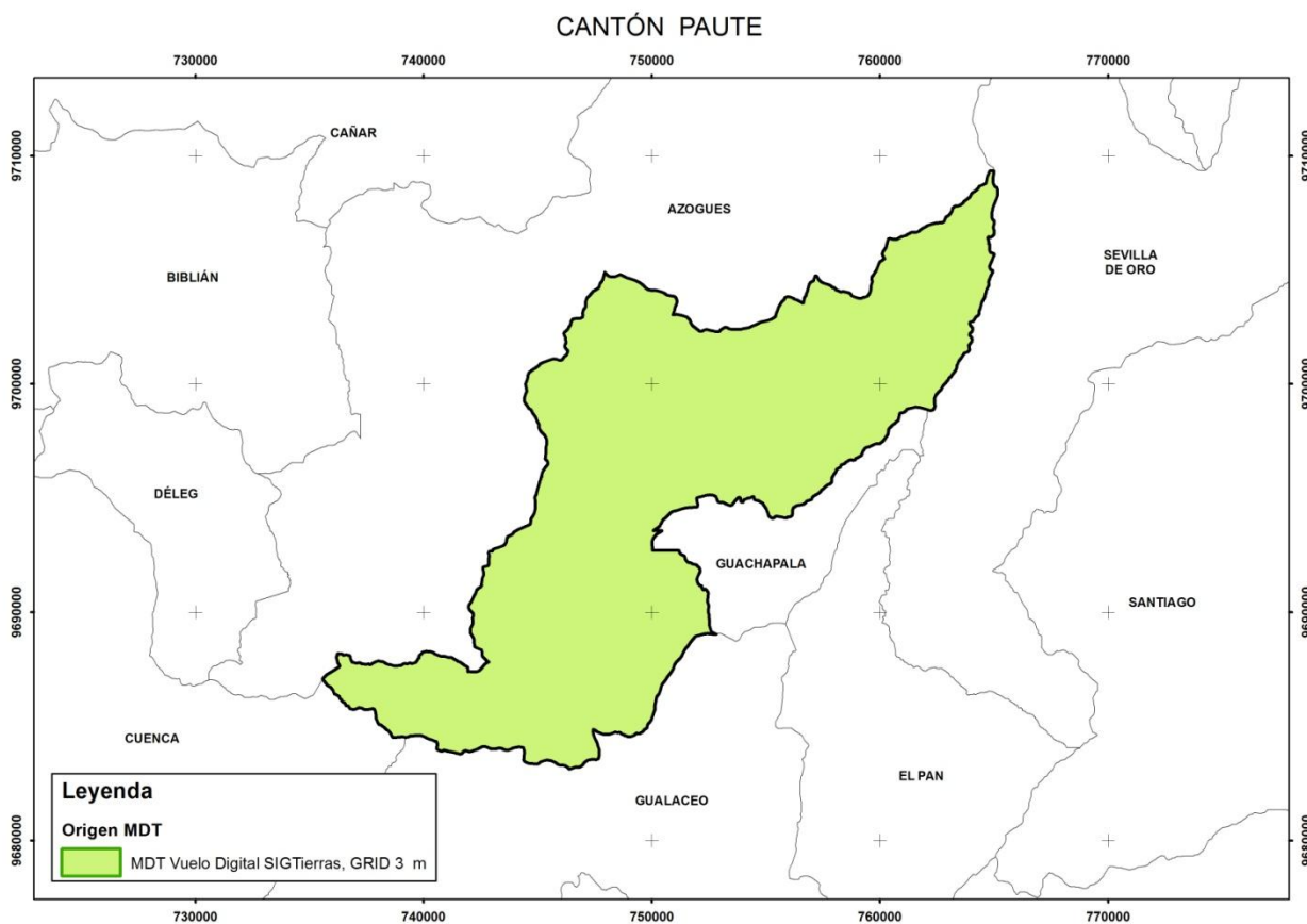
Figura 2.3. Insumos de base de generación de los MDT en el cantón Paute.
