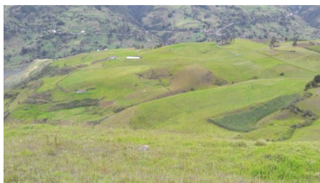
Fotos 4 y 5. Testigo de cono de esparcimiento. Sector Loma Shulunllún. 09/04/2014.
