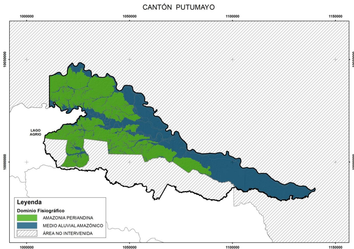
Figura 3.2. Distribución geográfica de los diferentes dominios fisiográficos presentes en el cantón Putumayo.
