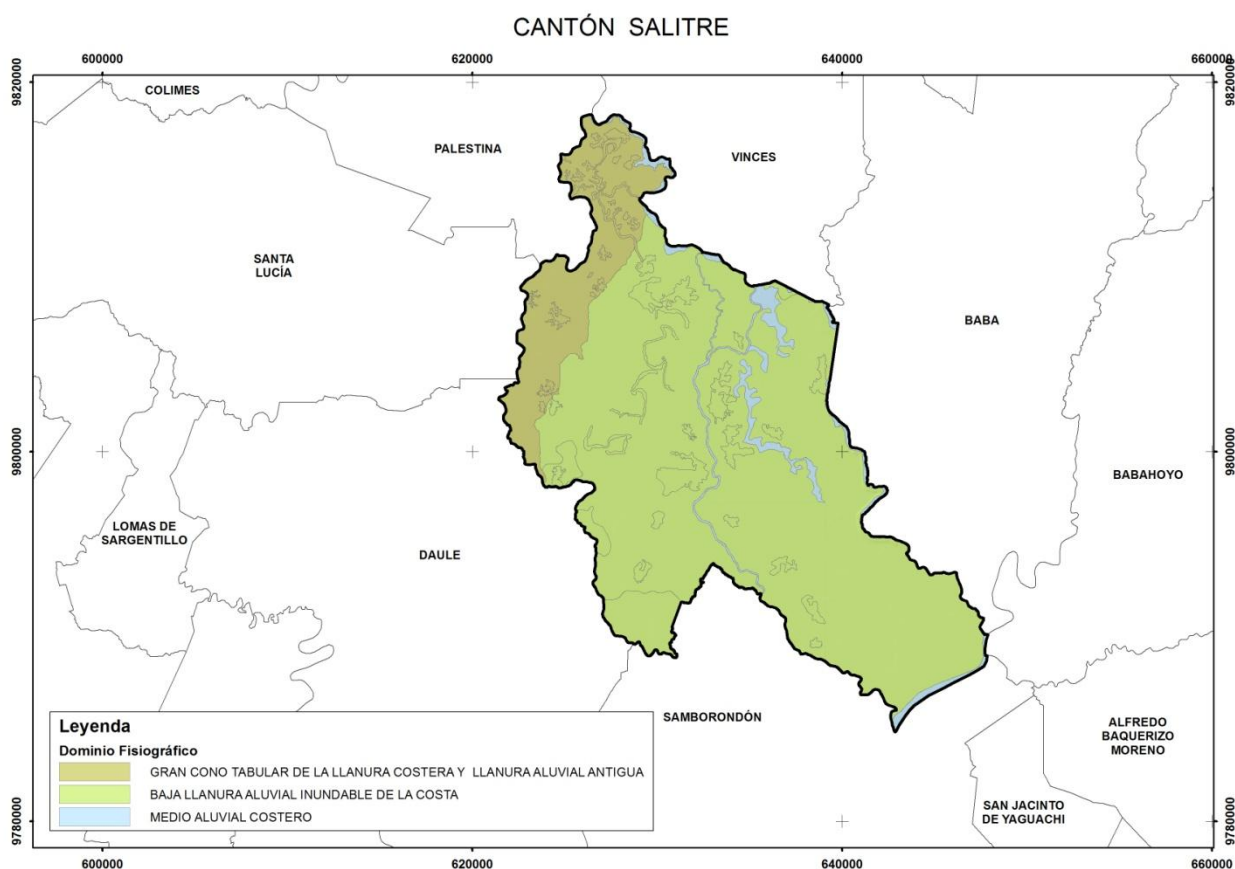
Figura 3.2. Distribución geográfica de los diferentes dominios fisiográficos presentes en el cantón Salitre.
