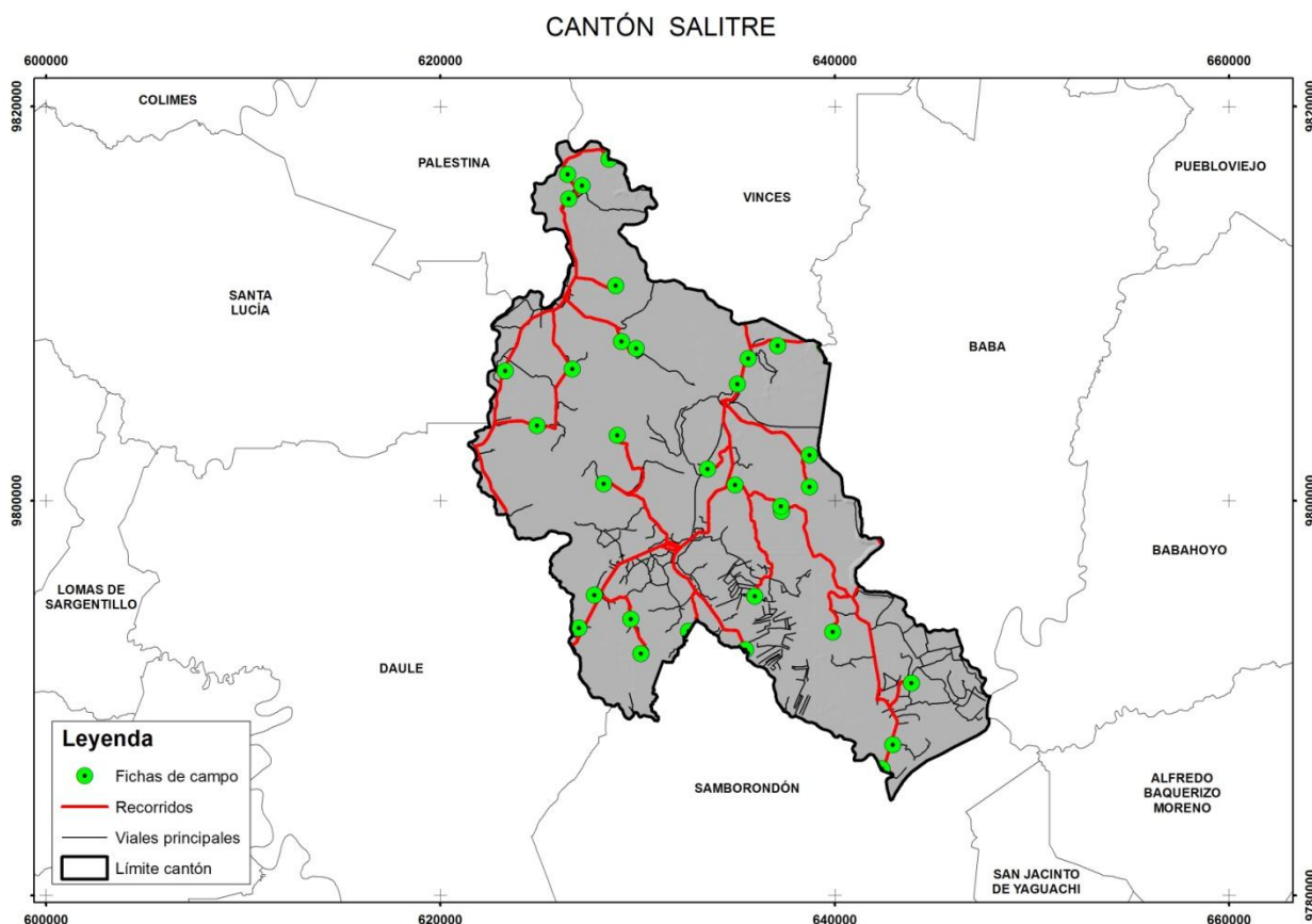
Figura 3.1. Localización de recorridos y fichas de campo del cantón Salitre.
