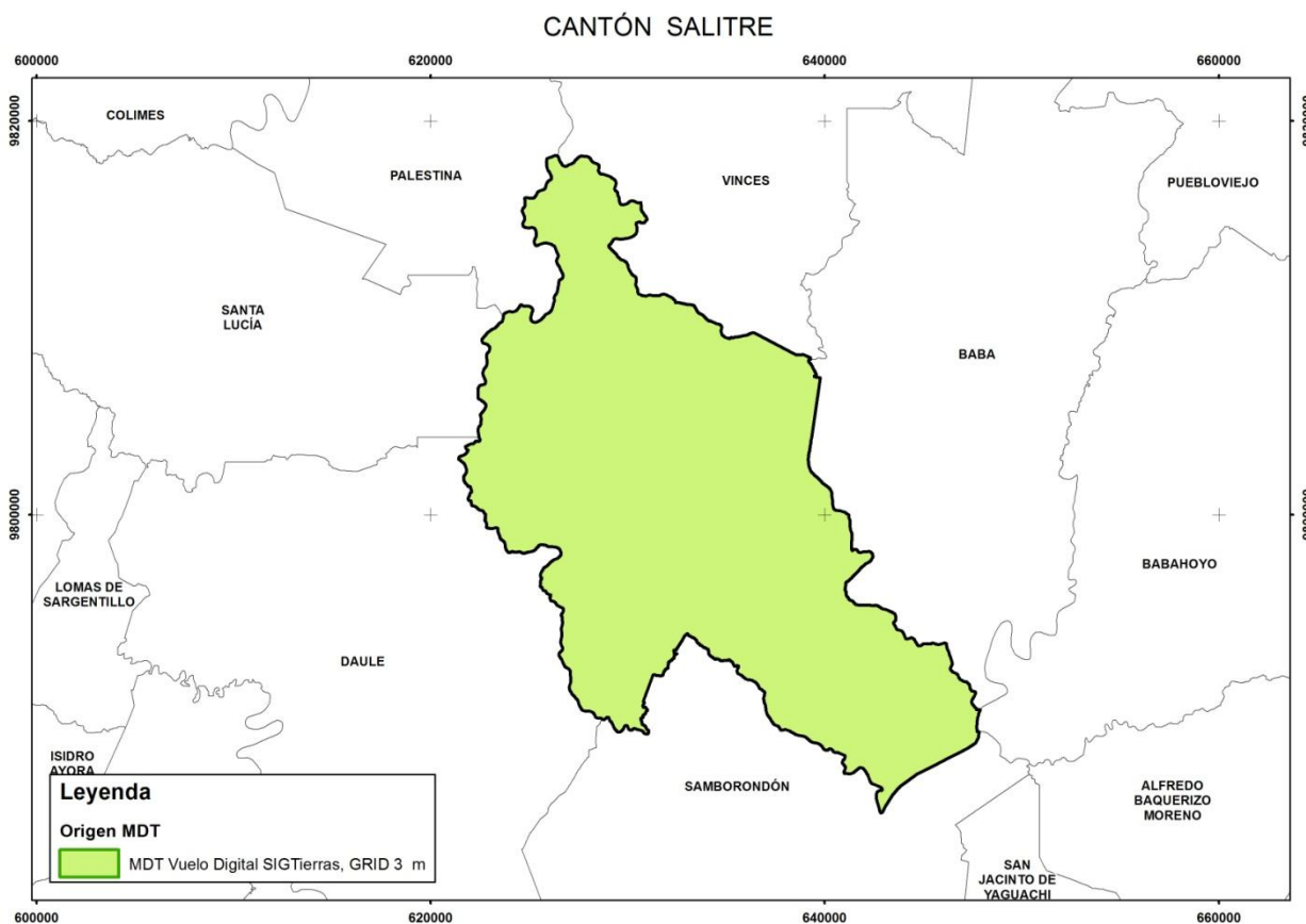
Figura 2.3. Insumos de base de generación de los MDT en el cantón Salitre.
