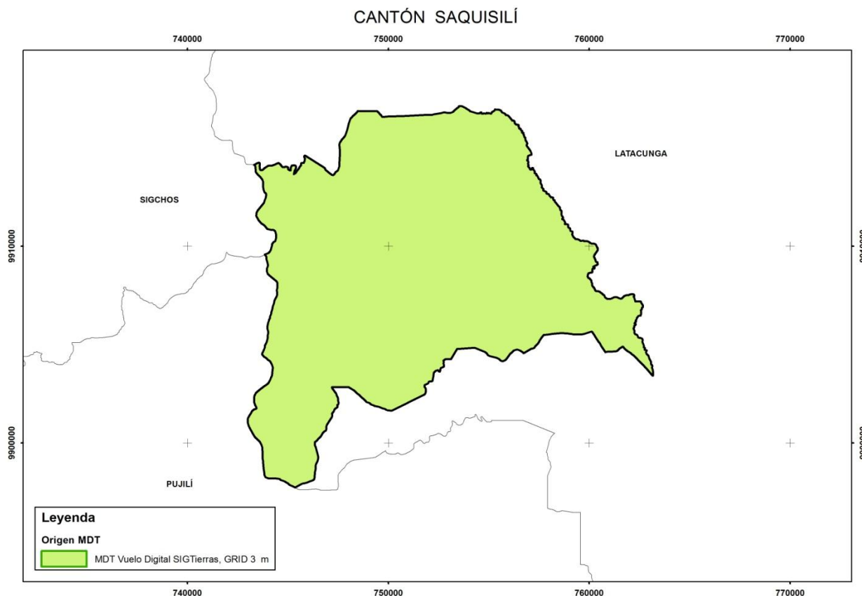
Figura 2.3. Insumos de base de generación de los MDT en el cantón Saquisilí.
