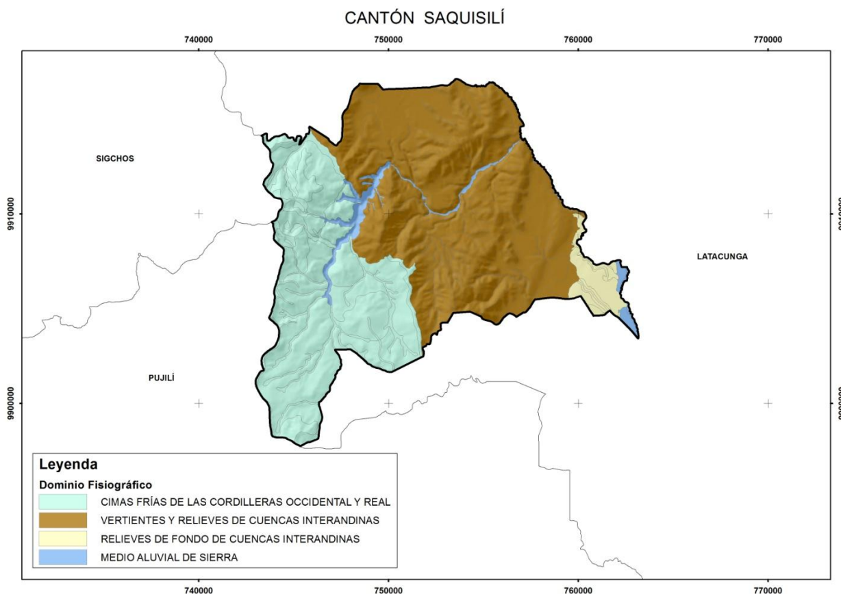
Figura 3.2. Distribución geográfica de los diferentes dominios fisiográficos presentes en el cantón Saquisilí.
