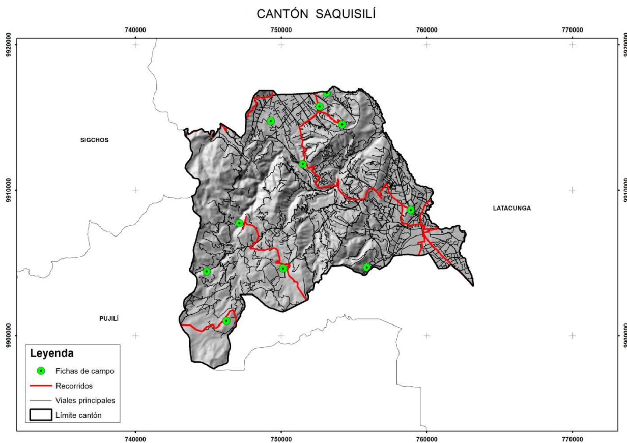
Figura 3.1. Localización de recorridos y fichas de campo del cantón Saquisilí.
