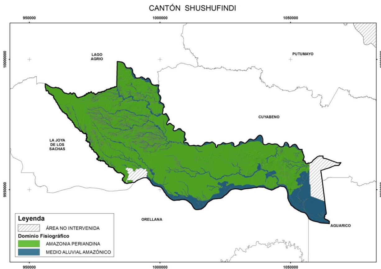
Figura 3.2. Distribución geográfica de los diferentes dominios fisiográficos presentes en el cantón Shushufindi.
