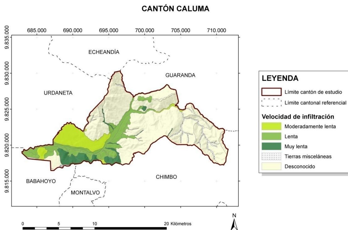
Figura 4.2 Mapa de Velocidad de infiltración determinada en los suelos del cantón Caluma
