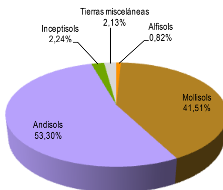
Gráfico 3.1 Representación de la distribución porcentual de los órdenes de suelos en el cantón Caluma
