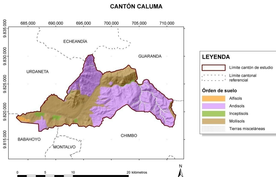
Figura 3.3. Ubicación de los diferentes órdenes de suelos en el cantón Caluma
