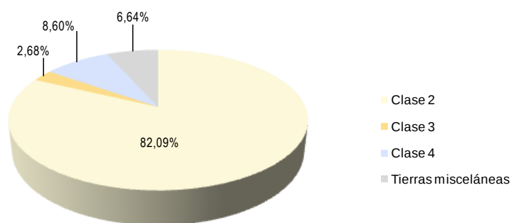
Gráfico 6.1. Representación de la distribución porcentual de las diferentes clases de dificultad de labranza de los suelos en el cantón Cevallos
