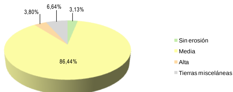
Gráfico 7.1. Representación de la distribución porcentual de las diferentes clases de amenaza a erosión hídrica en el cantón Cevallos
