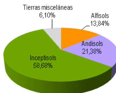
Gráfico 3.1 Representación de la distribución porcentual de los órdenes de suelos en el cantón Chilla
