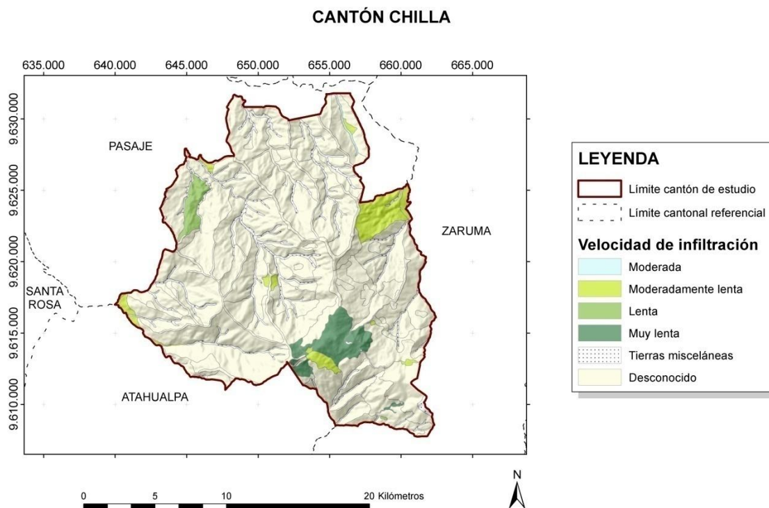
Figura 4.2 Mapa de Velocidad de infiltración determinada en los suelos del cantón Chilla
