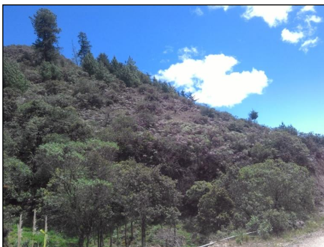
Foto 7.3. Zonas con amenaza Muy Alta a erosión hídrica en el cantón
