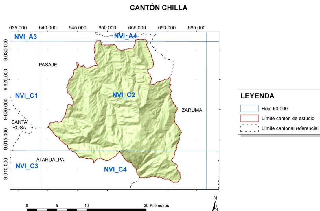
Figura 3.1. Ubicación del cantón Chilla en relación a las hojas topográficas del IGM, escala 1:50.000
