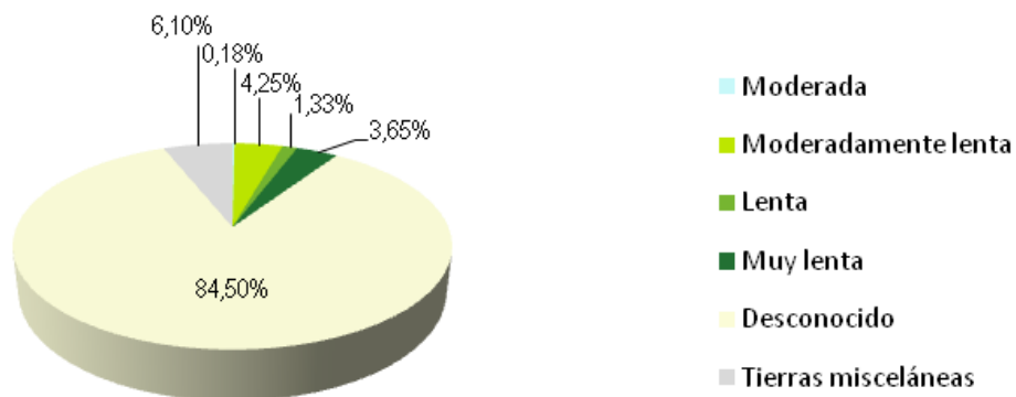
Gráfico 4.1. Distribución porcentual de las clases de Velocidad de infiltración de los suelos en el cantón Chilla
