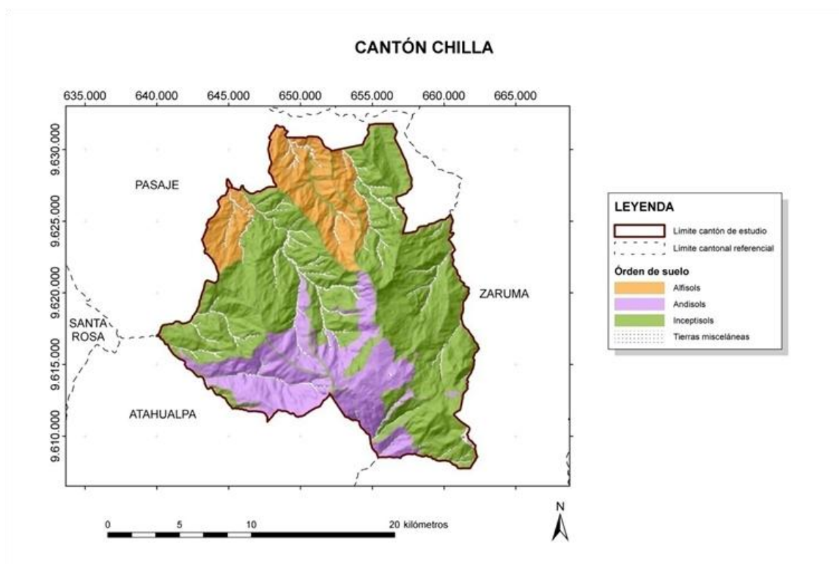
Figura 3.3. Ubicación de los diferentes órdenes de suelos en el cantón Chilla
