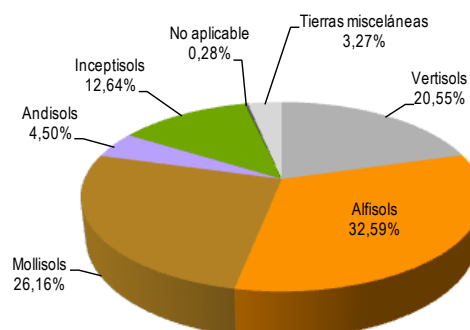
Gráfico 3.1 Representación de la distribución porcentual de los órdenes de suelos en el cantón Guachapala.
