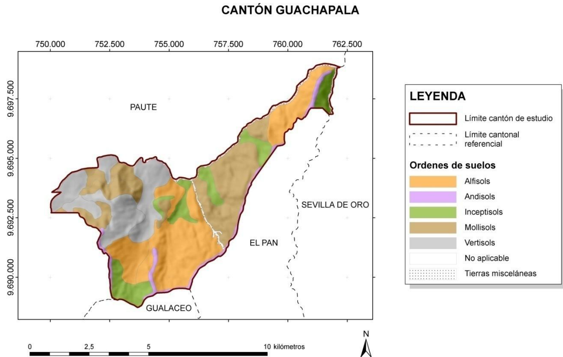
Figura 3.3. Ubicación de los diferentes órdenes de suelos en el cantón Guachapala.
