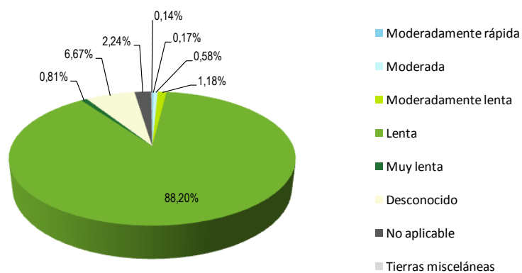
Gráfico 4.1. Distribución porcentual de las clases de Velocidad de infiltración de los suelos en el cantón La Troncal
