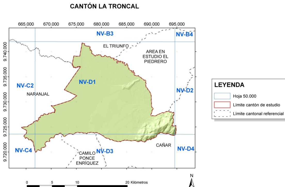
Figura 3.1. Ubicación del cantón La Troncal en relación a las hojas topográficas del IGM, escala 1:50.000
