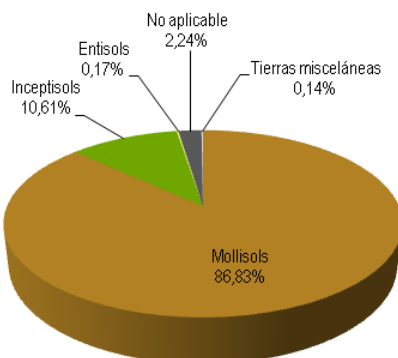
Gráfico 3.1 Representación de la distribución porcentual de los órdenes de suelos en el cantón La Troncal
