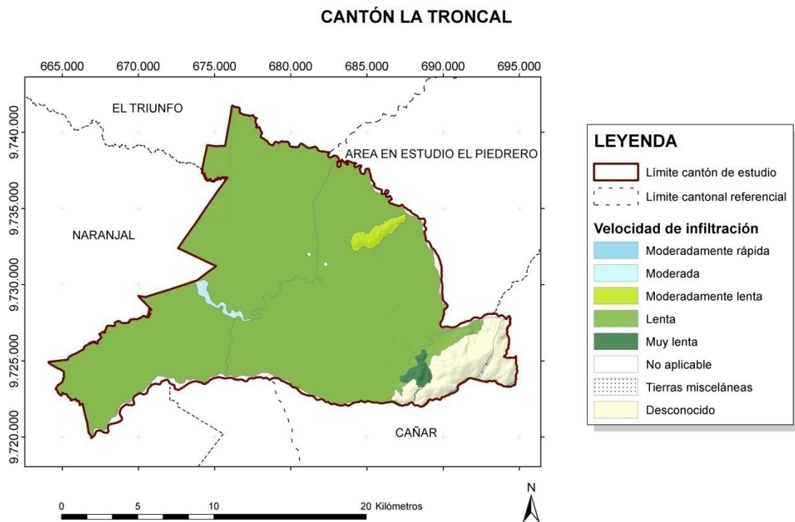
Figura 4.2 Mapa de Velocidad de infiltración determinada en los suelos del cantón La Troncal
