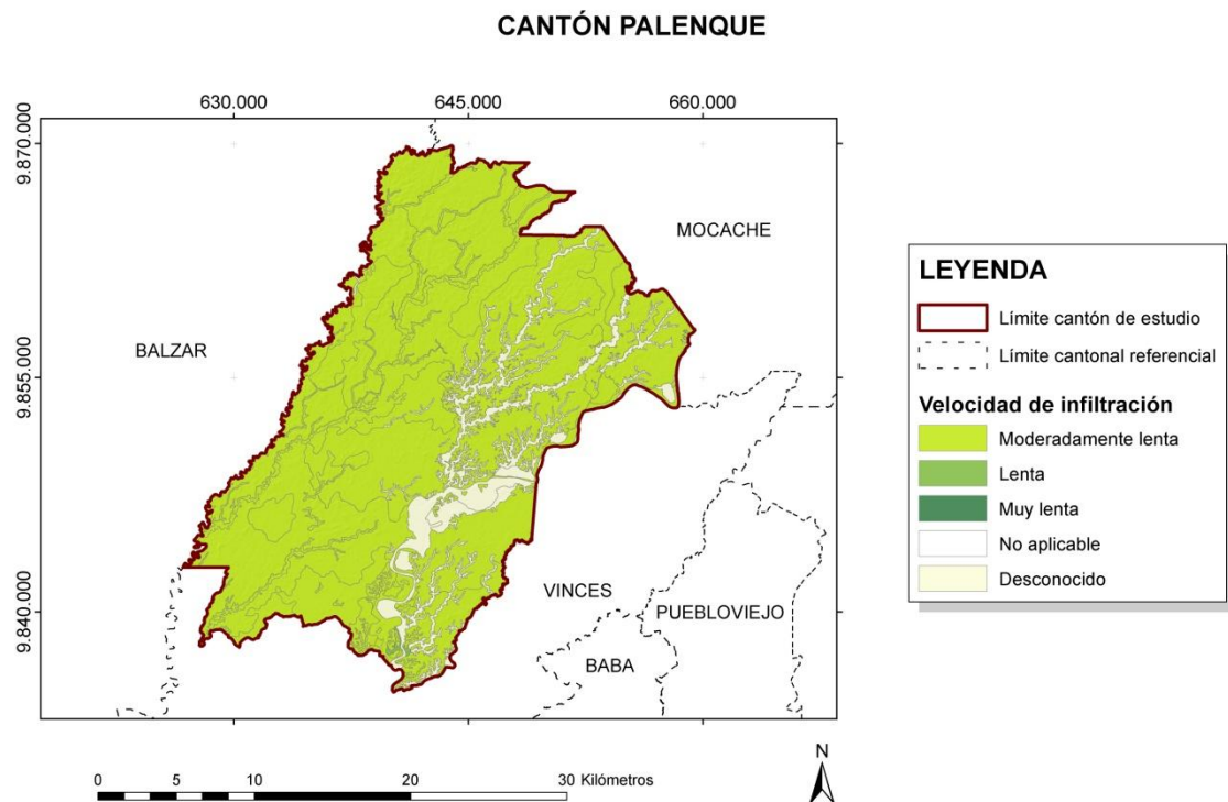
Figura 4.2 Mapa de Velocidad de infiltración determinada en los suelos del cantón Palenque
