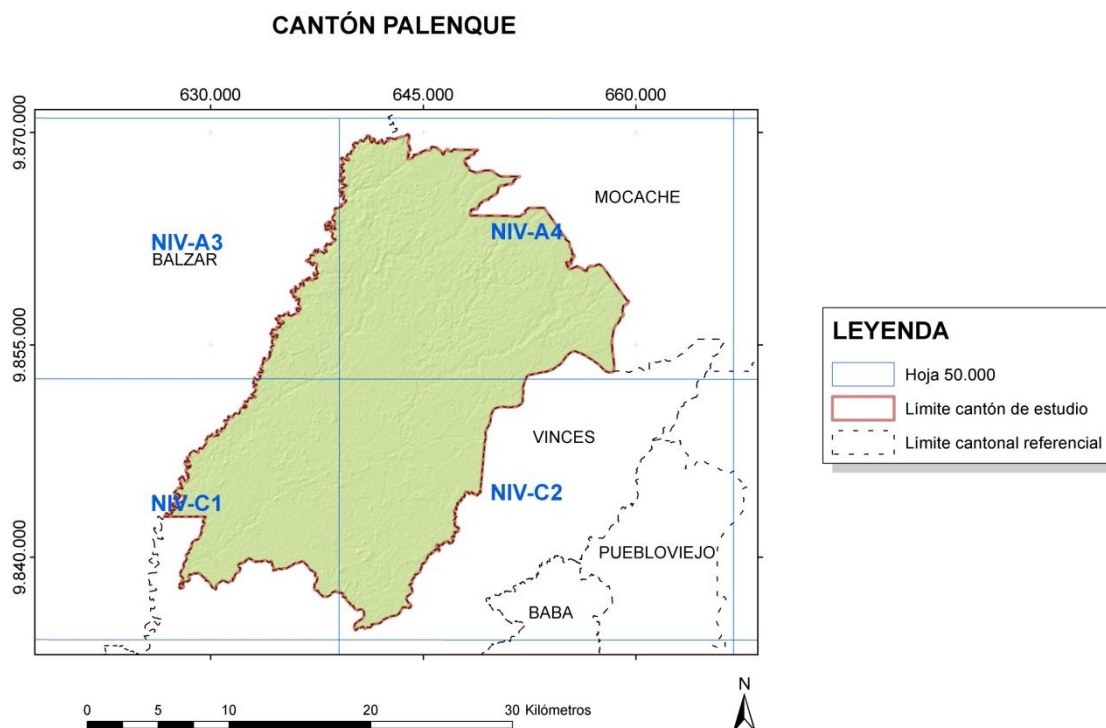
Figura 3.1. Ubicación del cantón Palenque en relación a las hojas topográficas del IGM, escala 1:50.000
