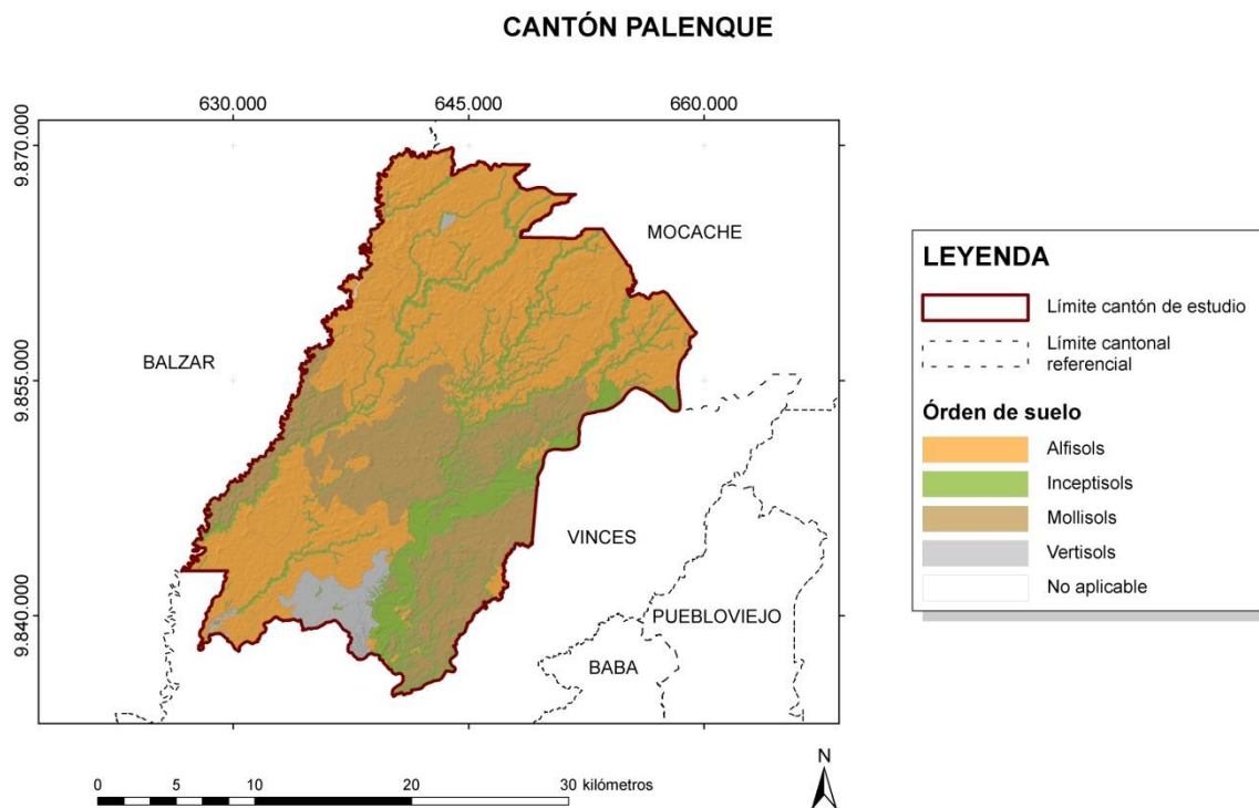
Figura 3.3. Ubicación de los diferentes órdenes de suelos en el cantón Palenque
