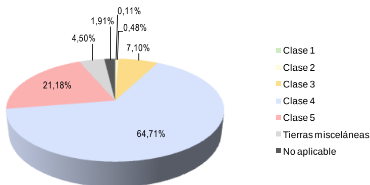
Gráfico 6.1. Representación de la distribución porcentual de las diferentes clases de dificultad de labranza de los suelos en el cantón
