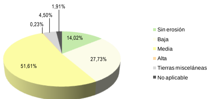
Gráfico 7.1. Representación de la distribución porcentual de las diferentes clases de amenaza a erosión hídrica en el cantón
