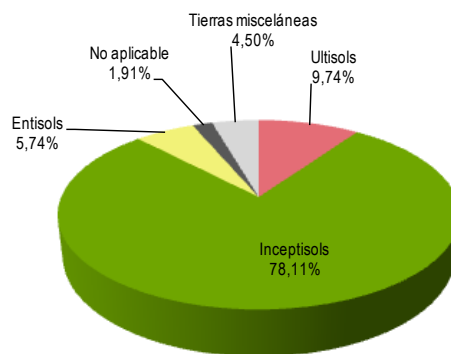
Gráfico 3.1 Representación de la distribución porcentual de los órdenes de suelos en el cantón Tiwintza
