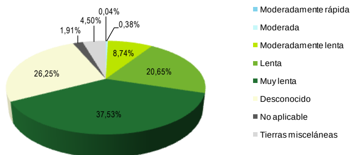
Gráfico 4.1. Distribución porcentual de las clases de Velocidad de infiltración de los suelos en el cantón Tiwintza
